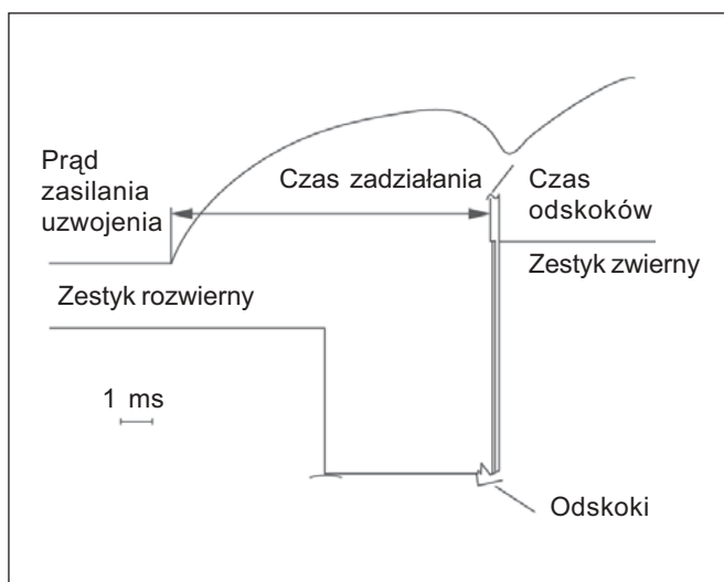
Rys. 25. Czas zadziałania
