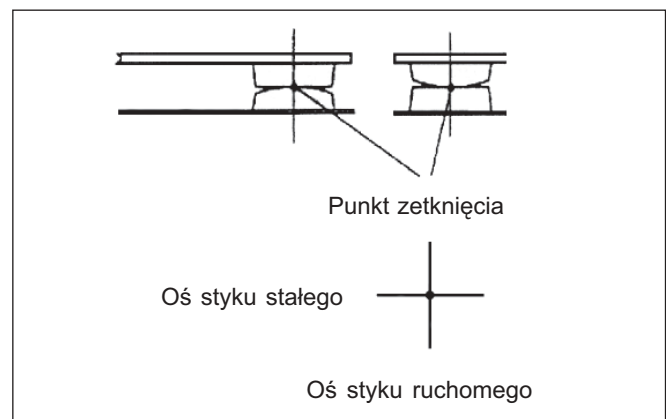
Rys. 15. Styk krzyżowy
