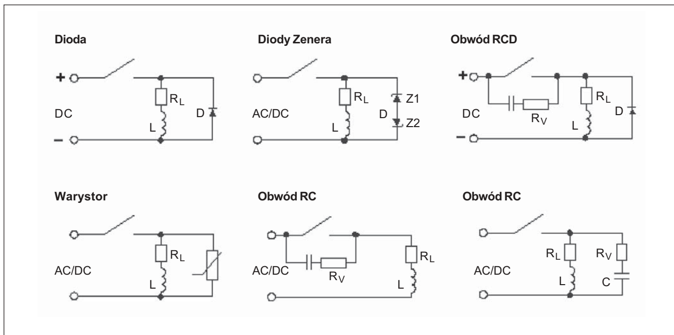
Rys. 23. Obwody zabezpieczające
