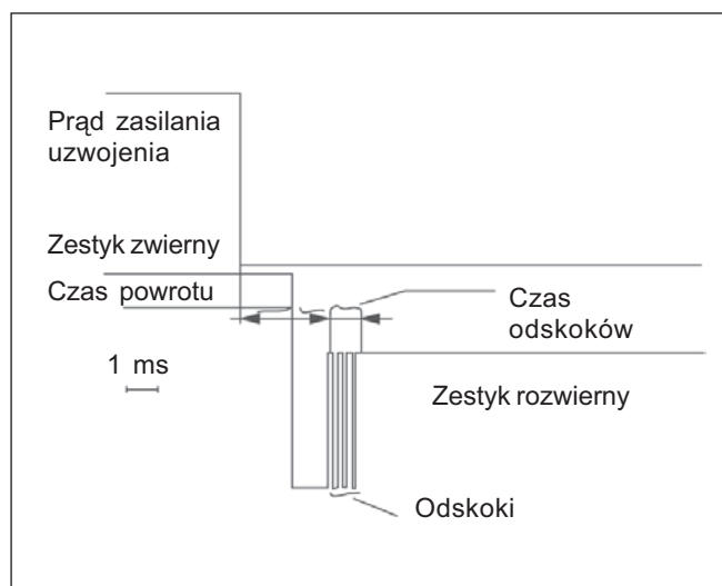
Rys. 26. Czas powrotu
