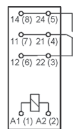
1P - przełączny
