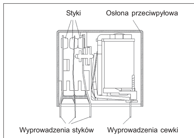
Rys. 2. Klasyczna budowa przełącznika
