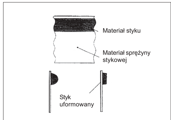
Rys. 14. Styk o małym profilu
