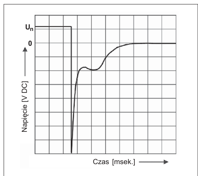
Rys. 9. Napięcie na cewce DC podczas wyłączania
