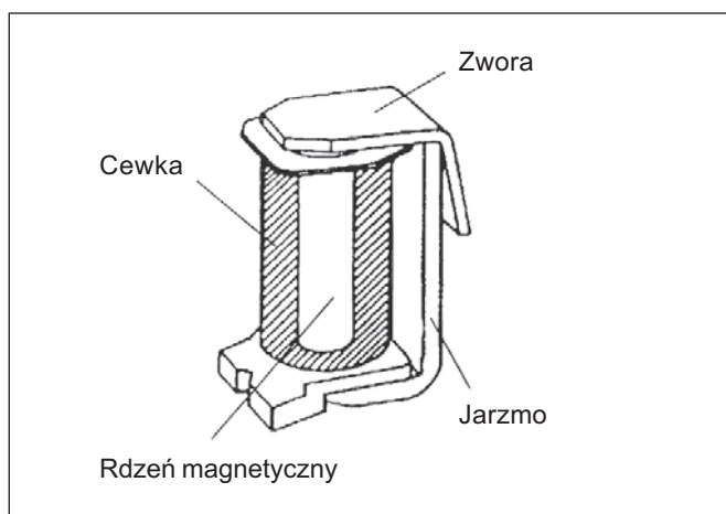
Rys. 1. Klasyczny układ elektromagnesu
