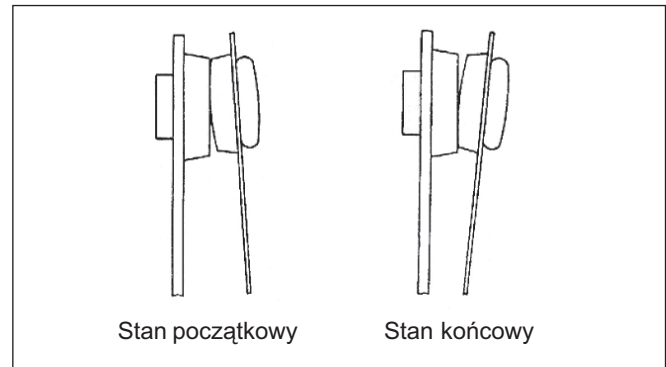
Rys. 13. Ruch styków
