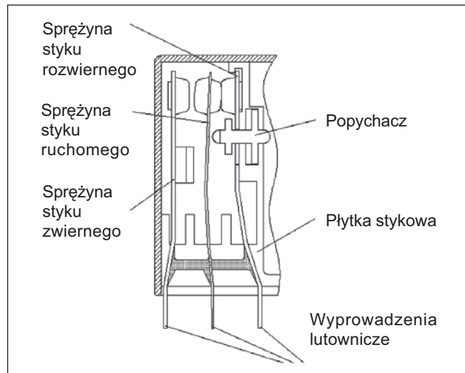
Rys. 3. Sekcja przełączania przełącznika
